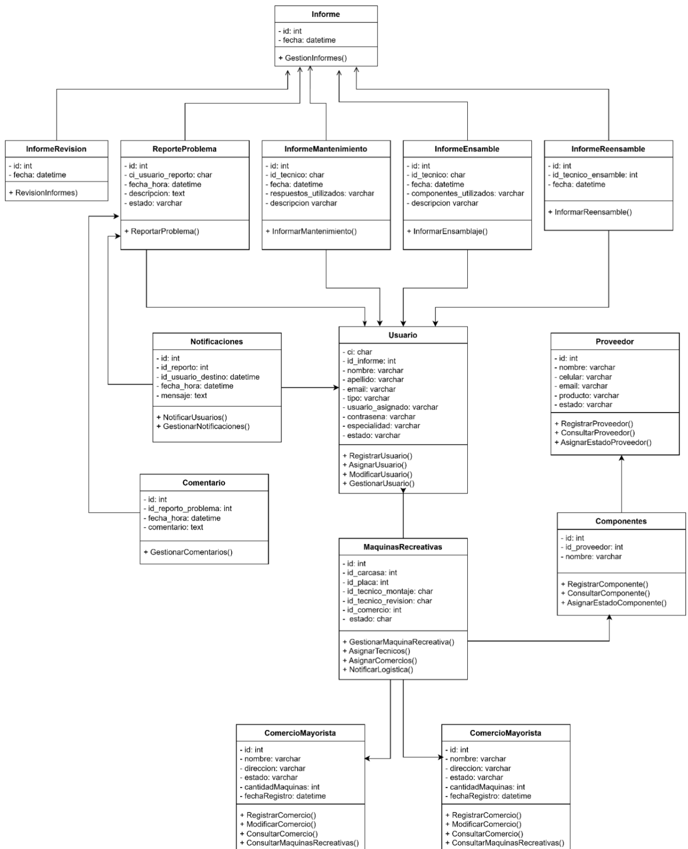
Diagrama de clases
