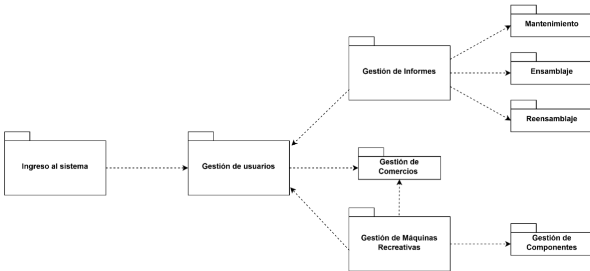
Diagrama de paquetes
